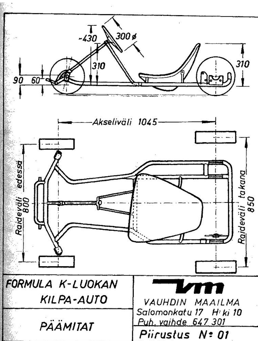
Formula K-luokan kilpa-auton eli Mäkäran akseliväli oli hiukan toista metriä. Piirokset julkaistiin aikoinaan Vauhdin Maailmassa.
